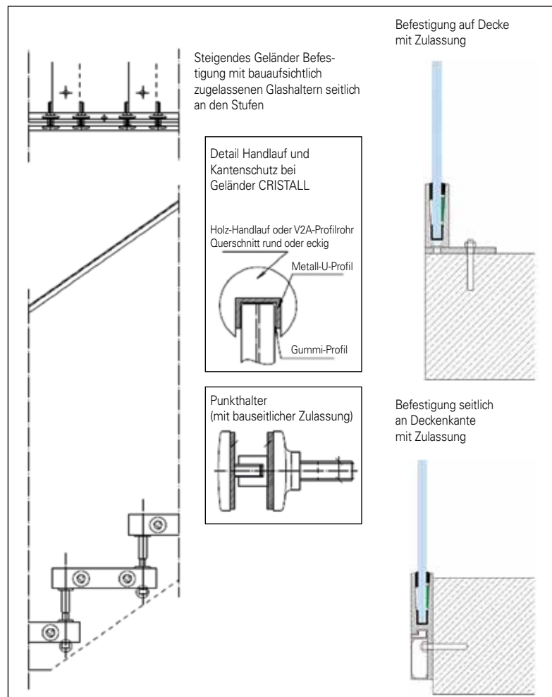
Seitlich befestigtes Ganzglasgeländer CRISTALL mit wählbarem Handlauf/ Kantenschutzprofil (Abb.-Beispiel)
